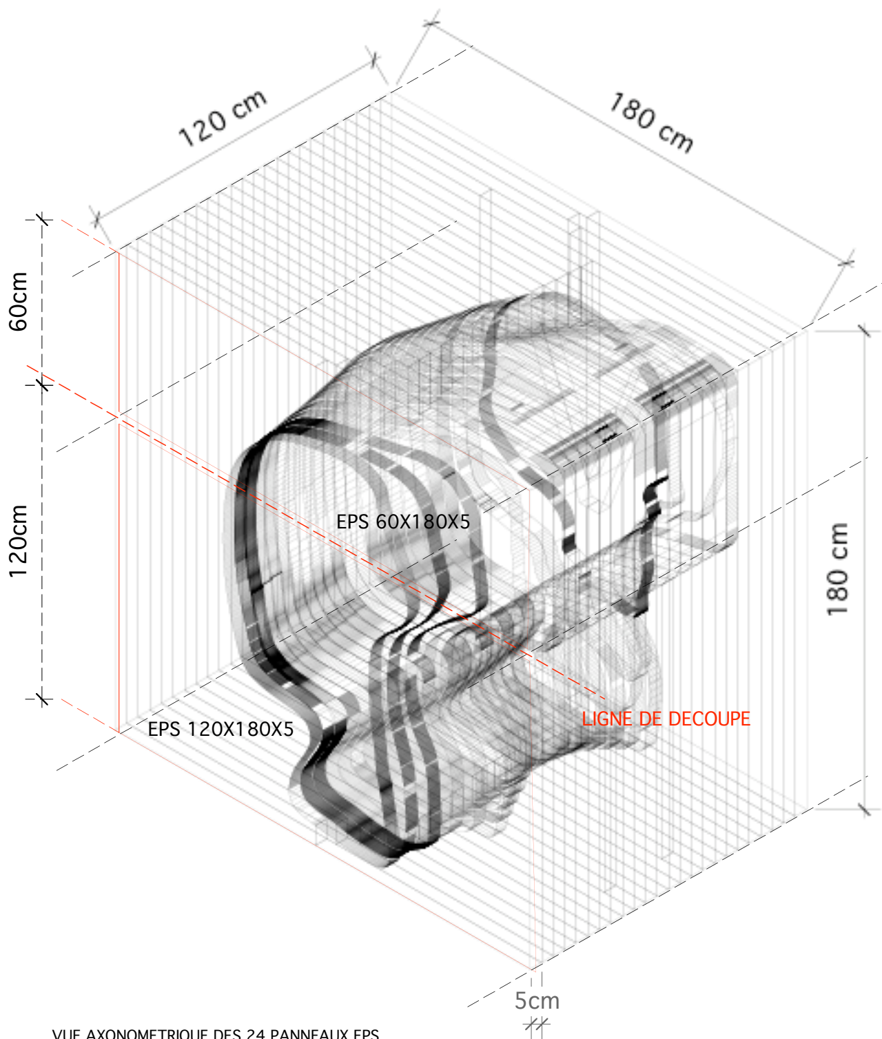
VUE AXONOMETRIQUE DES 24 PANNEAUX EPS (L: 5CM, D: 20KG/M3), COLLES APRES DECOUPE
